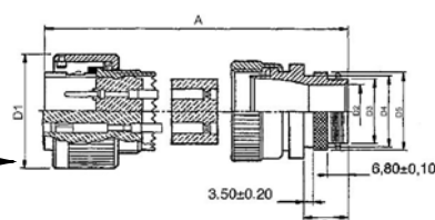
VG3106EW-B-TLXX 带记忆环的直式插头
