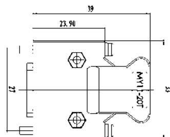
外形尺寸
