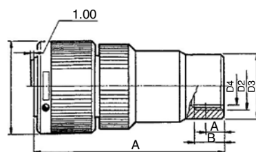
VG3106PG 带管制螺 纹的直式插头
