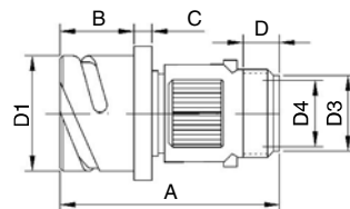
VG3101F 中继插座 (02、03、06)
