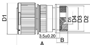
VG3106E 直式插头 (02、03、04)
