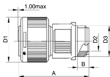
VG3106F 直式插头
