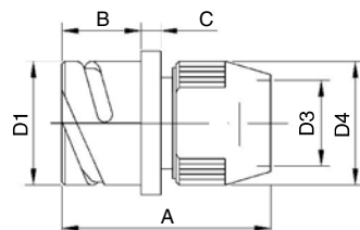
VG3101R 中继插座
