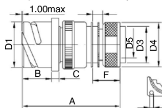
VG3100E 墙式 安装插座 (32、32-05 屏蔽)
