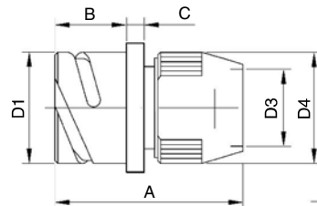
VG3100R 墙式 安装插座 (带短尾附)
