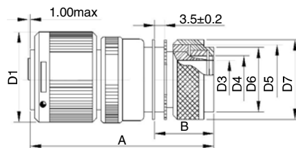
VG3106E 直式插头 (32、DXX)
