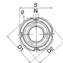
07A 螺母安装插座
