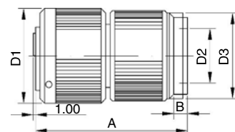
VG3106F 直式屏蔽插头 (13、14、15 可接波形管)
