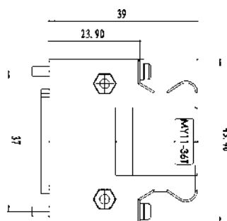
外形尺寸
