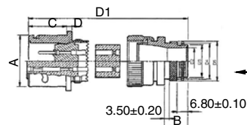
VG00EP-B-TLXX 带记忆环尾附件的 墙式安装插座
