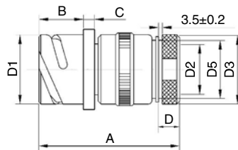
VG3101E 中继插座 (02、03、06)
