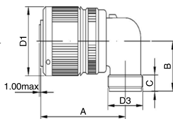
VG3108F 弯式屏蔽插头 (13、14、15 可接波 形管)
